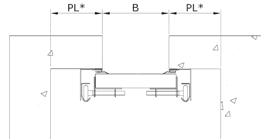
Vaakaleikkaus
