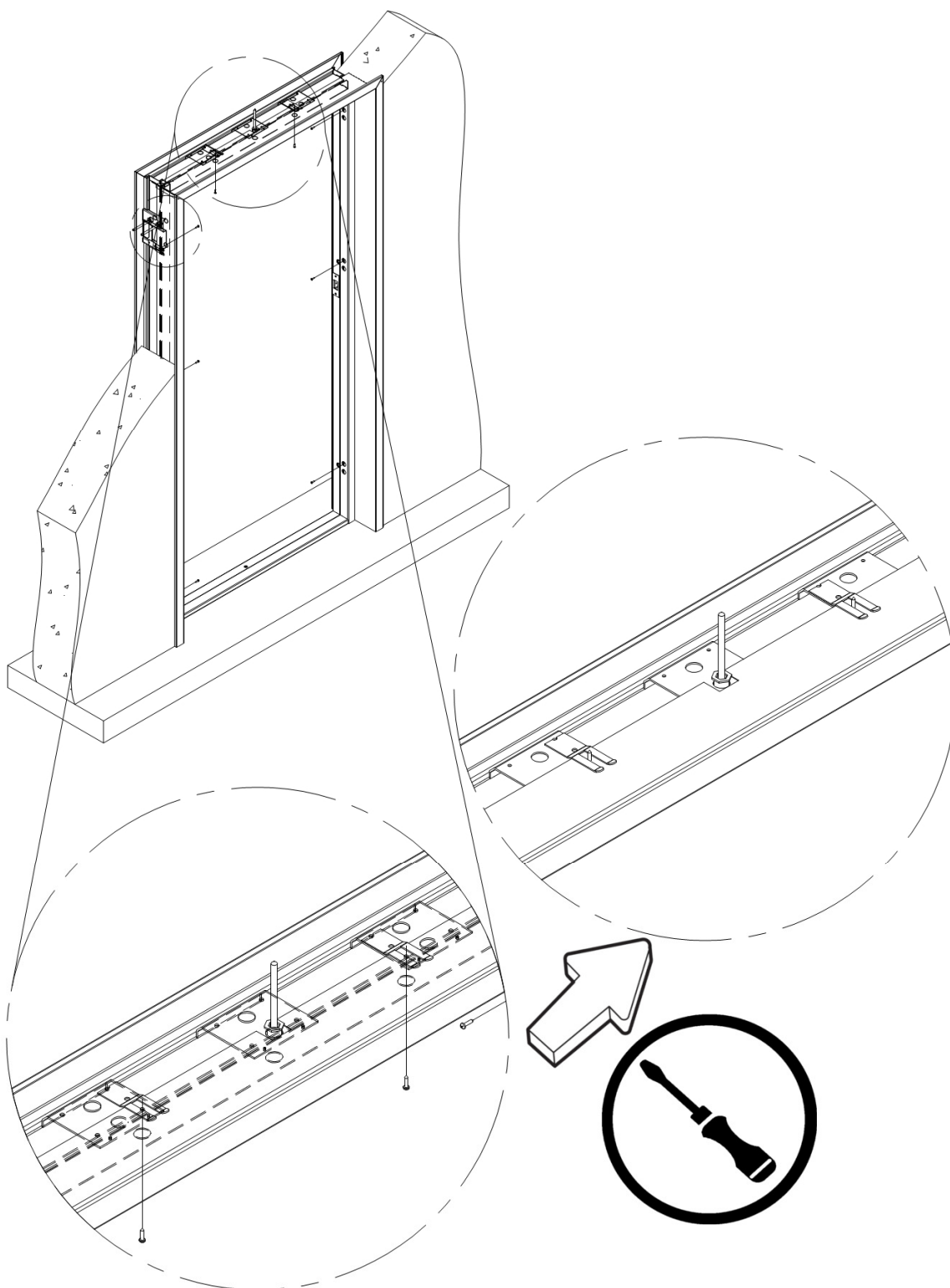
Kuva 2.5 Vastakappaleen kiinnittäminen karmiin.
