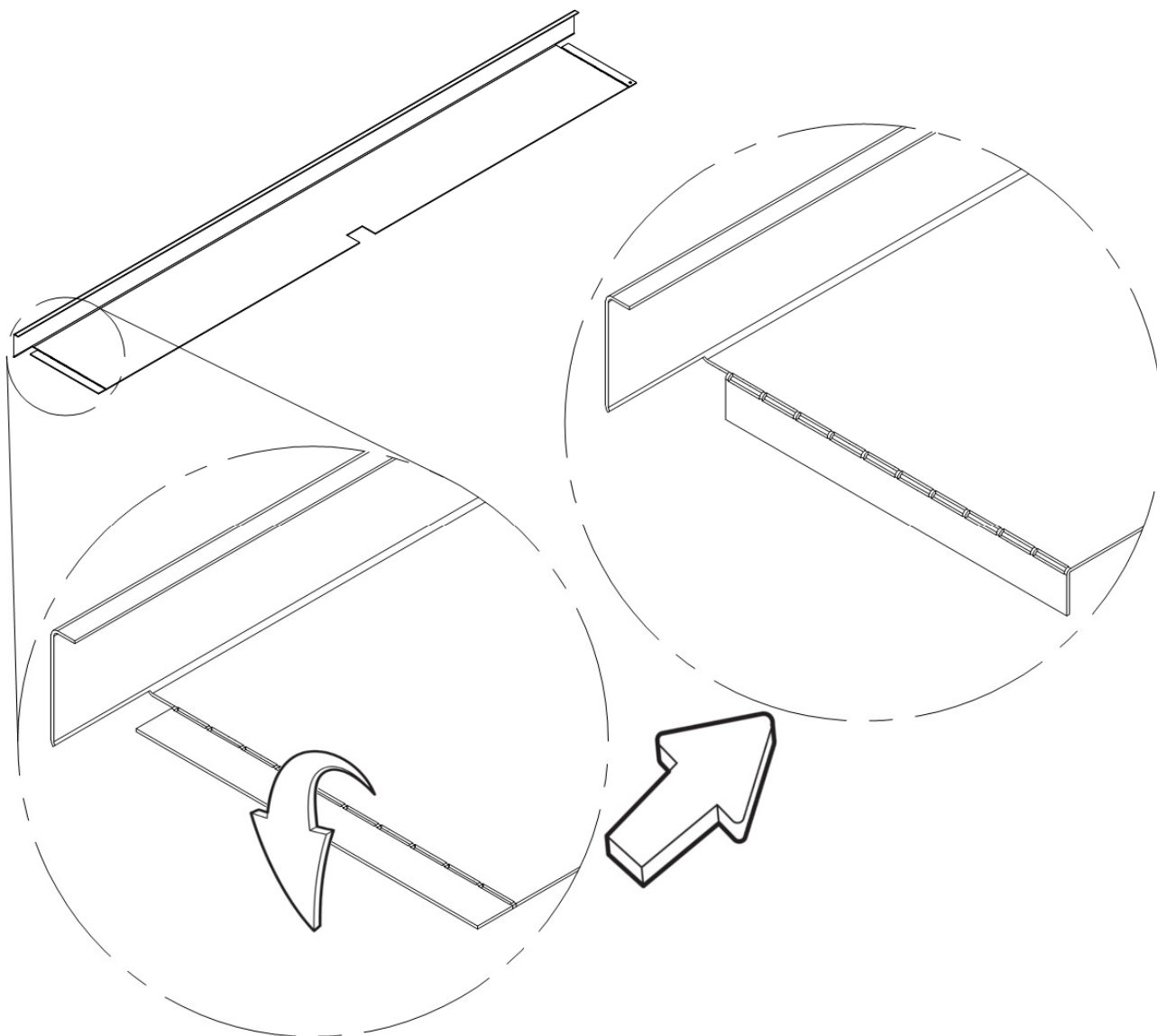
Kuva 2.2 Vastakappaleen yläosan taivutus.
