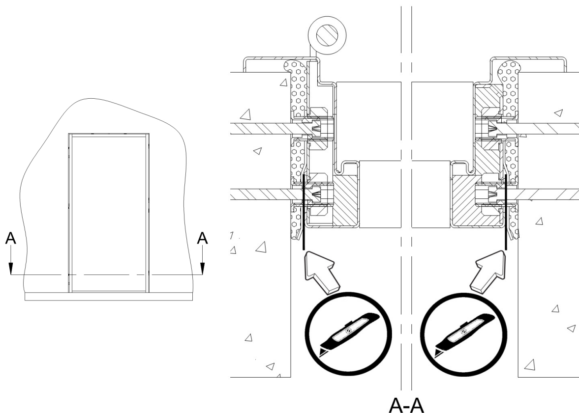
Kuva 2.1 Uran leikkaaminen karmin kehälle.
