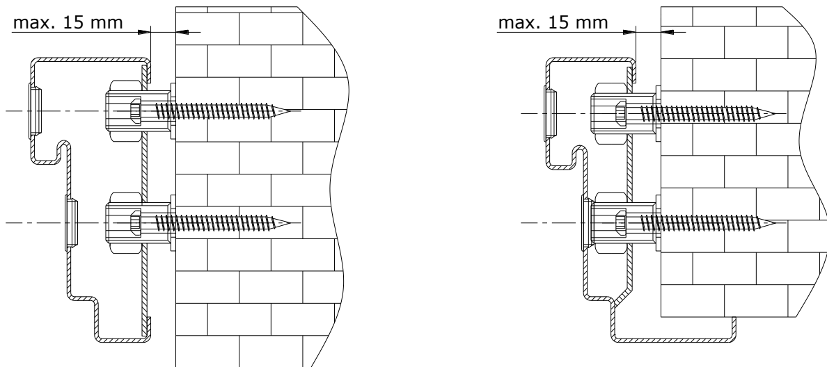
Piirros 3. Karmin kiinnitys holkkeilla
