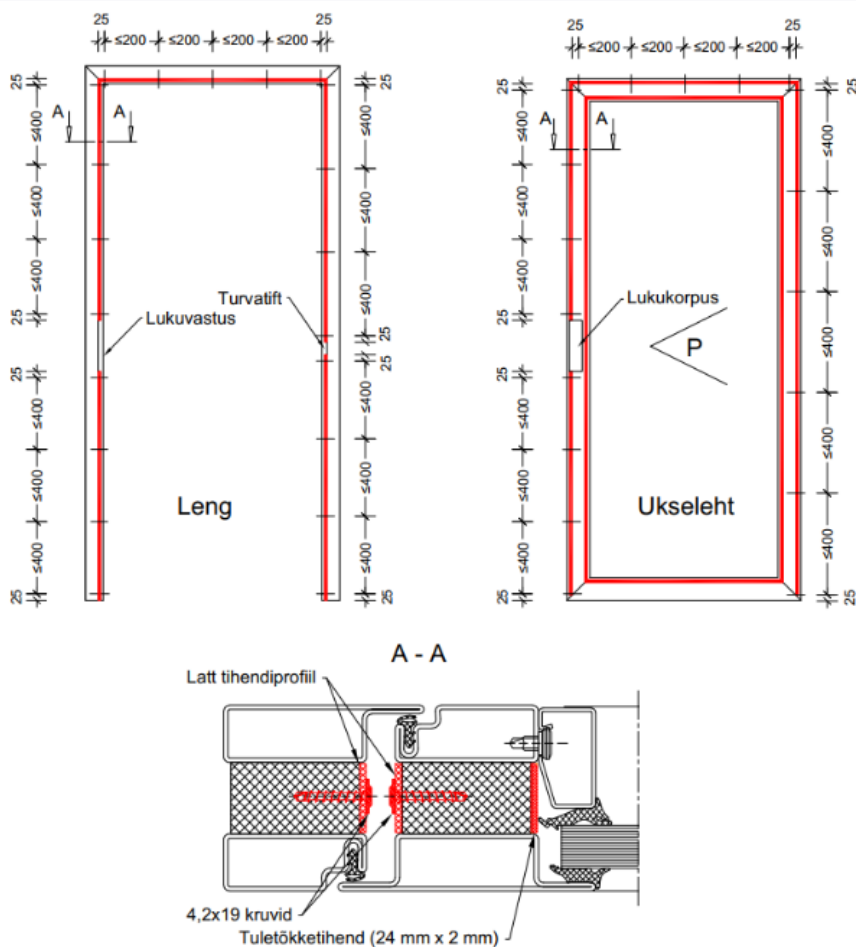
Joonis 4 Tuletõkketihendite paigaldus
