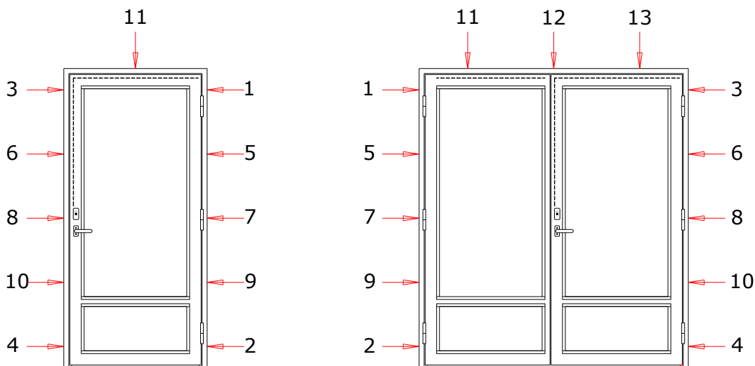
Joonis 3 Seinakinnituste järjekord uksele
