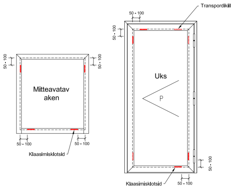
Joonis 9 Klaasimisklotside asukohad
