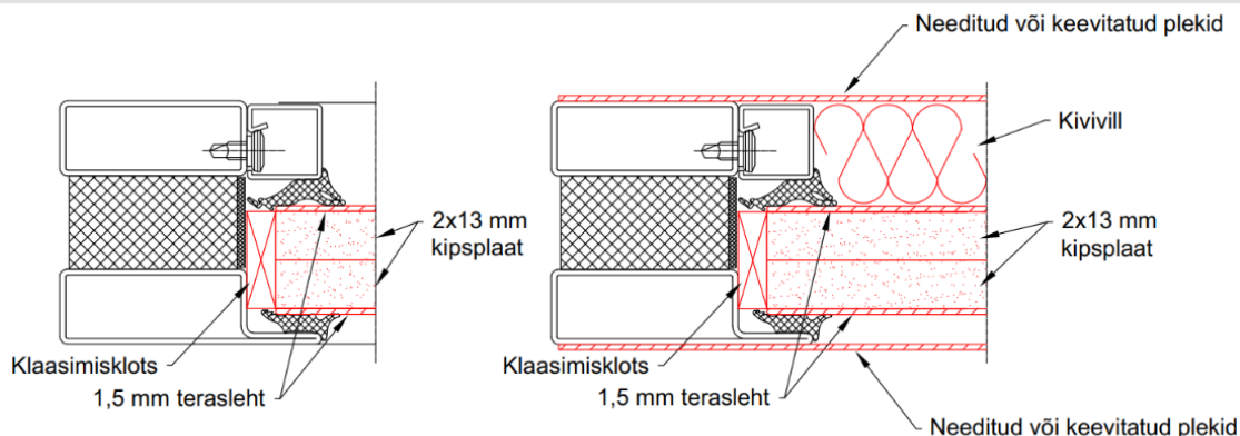
Joonis 8 Paneelide variandid EI30 tootele
