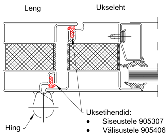
Joonis 5 Uksetihendite paigaldus
