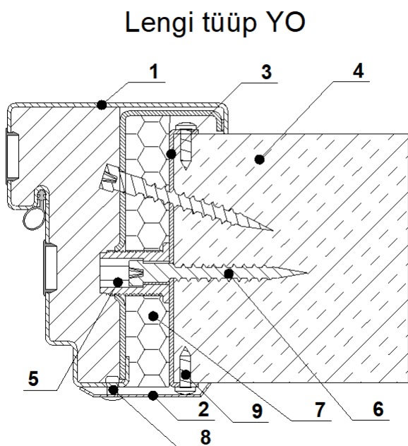
Joonis 3. Lengi kinnitus Sandwich- paneeli
